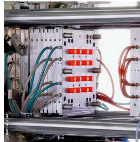
Blick in offenes Spritzguss-Produktionswerkzeug
